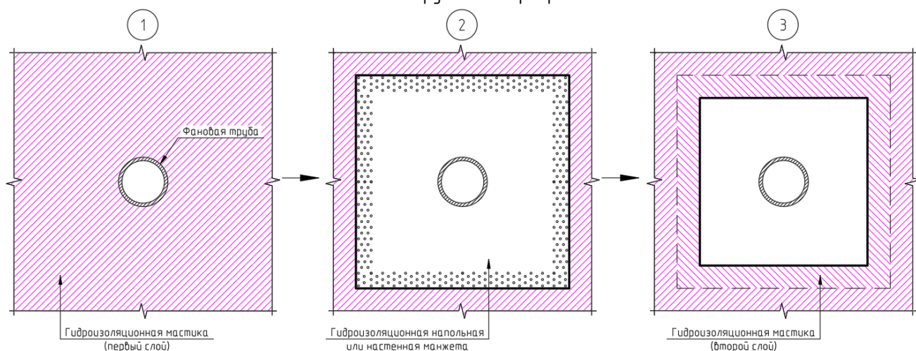
Рис.28. Последовательность нанесения гидроизоляционной манжеты.
