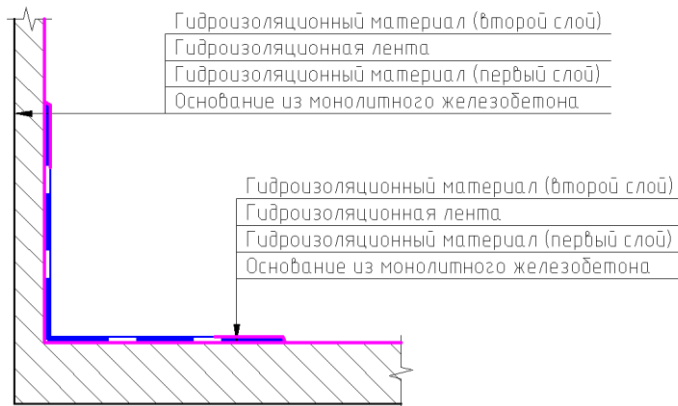
Рис.24. Устройство гидроизоляции внутренних углов с применением «PLITONIT ГидроЛента» и «PLITONIT ГидроЛента угол внутренний 90°».
