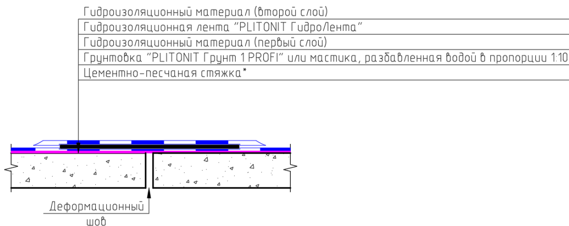
Рис.27. Конструктивный разрез №7.
