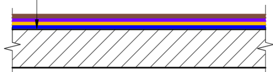
Рис.23. Конструктивный разрез №4.
