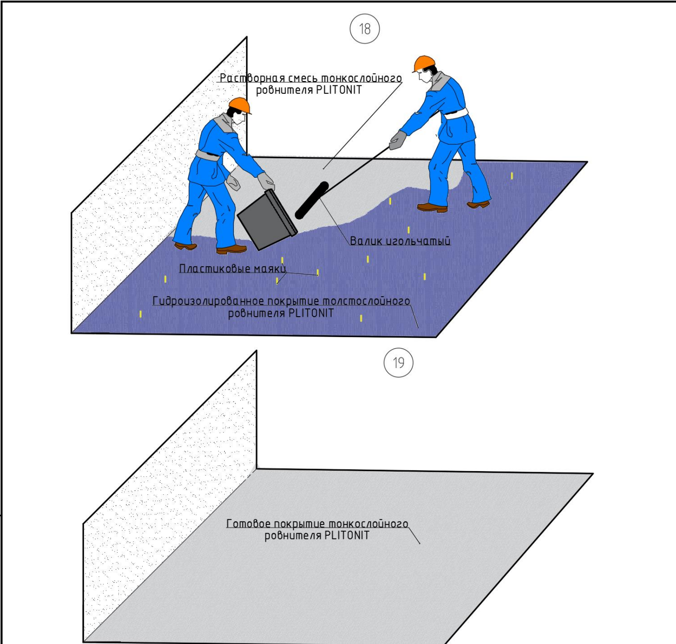
Рис.31. Последовательность работ, где: 1 – расправка грунтовки PLITONIT; 2 – перемешка грунтовки PLITONIT; 3 – нанесение грунтовки PLITONIT; 4 – подготовка покрытия к укладке толстослойного ровнителя PLITONIT; 5 – приготовление смеси толстослойного ровнителя PLITONIT; 6-7– укладка толстослойного ровнителя PLITONIT; 8 – готовое покрытие толстослойного ровнителя PLITONIT; 9 – расправка грунтовки PLITONIT; 10 – перемешка грунтовки PLITONIT; 11 – нанесение грунтовки PLITONIT; 12 – укладка гидроизоляционной ленты на поверхность, предварительно обработанную «PLITONIT ГидроЭласт»; 13 – поверхностная обработка ленты гидроизоляцией «PLITONIT ГидроЭласт»; 14 – нанесение первого слоя гидроизоляции на основание (горизонтальное); 15 – нанесение последующего слоя гидроизоляции на основание (горизонтальное); 16 – подготовка покрытия к укладке тонкослойного ровнителя PLITONIT; 17 – приготовление смеси тонкослойного ровнителя PLITONIT; 18– укладка тонкослойного ровнителя PLITONIT; 19 – готовое покрытие тонкослойного ровнителя PLITONIT.
